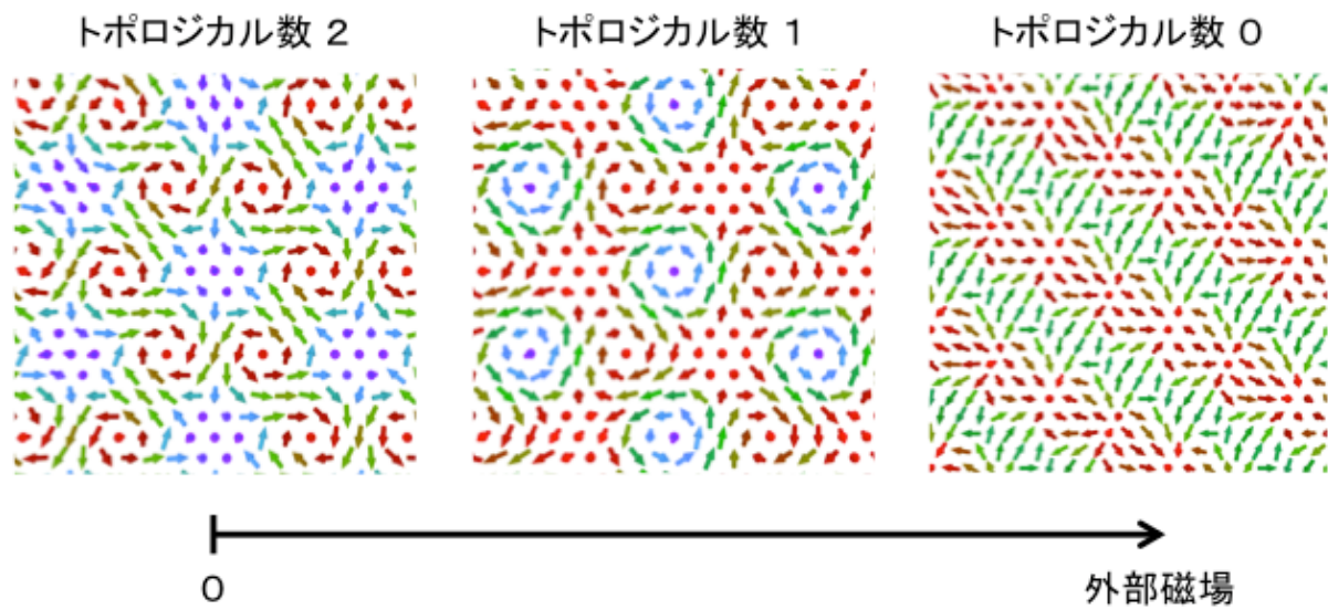
図 3：磁場によるトポロジカル数の多段階変化
