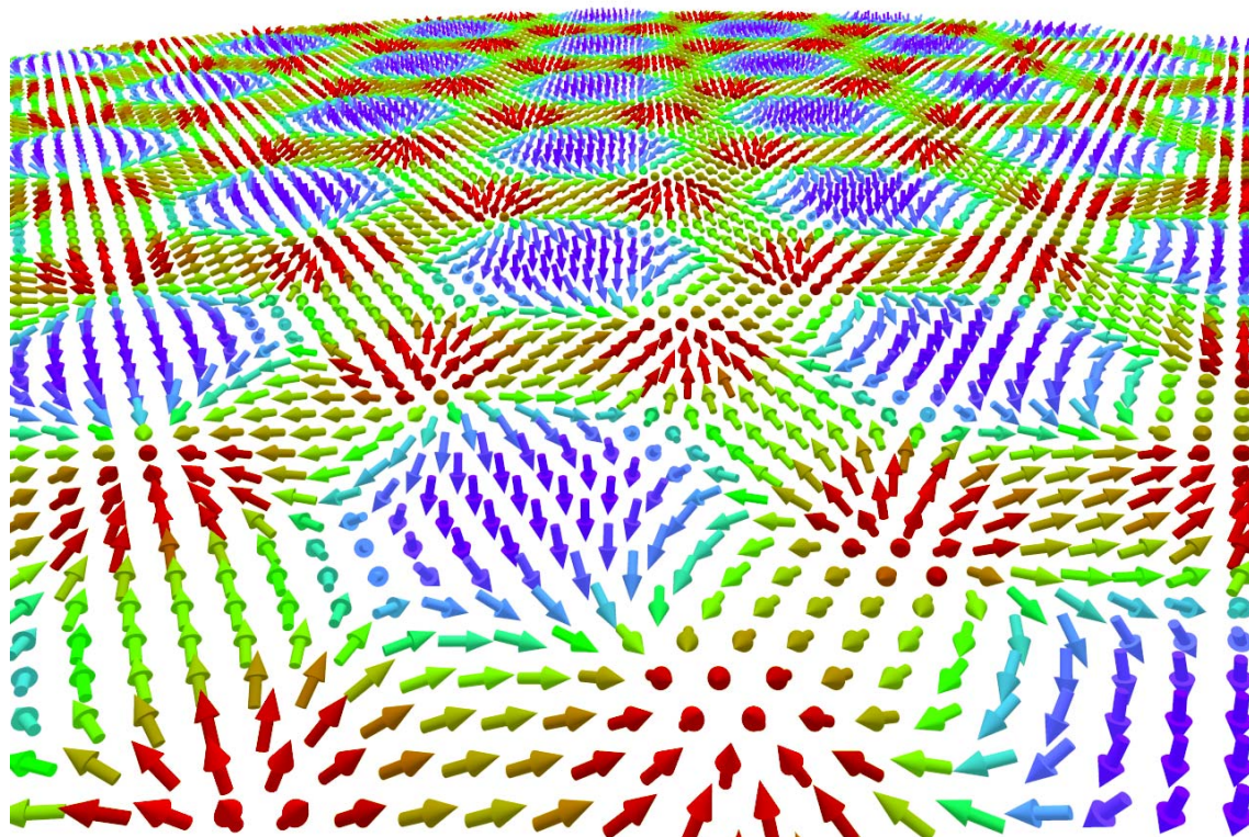
図2：トポロジカル数2の磁気スキルミオン結晶の模式図
