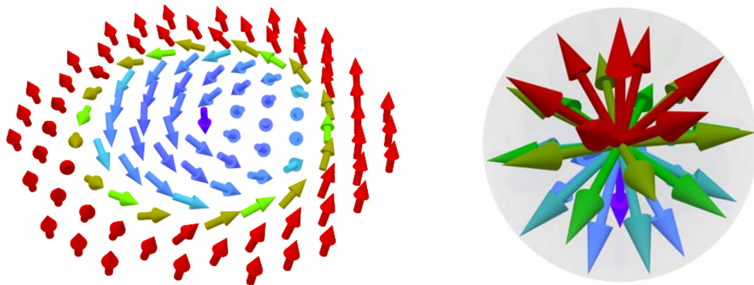
図1：磁気スキルミオンの概念図
