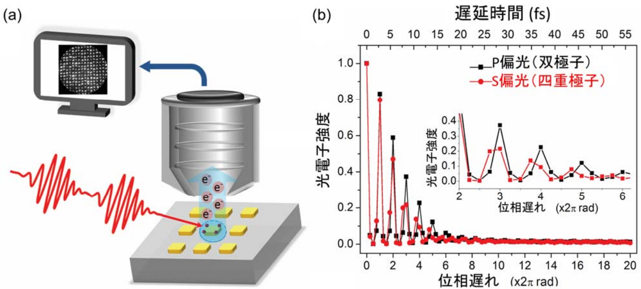
図2 (a) 金ナノ微粒子から飛び出した電子を高分解能で画像化できる顕微鏡にレーザー光線を2つの光線に分割し、2つ目の光線を時間遅延させることにより、コマ撮り写真の要領で電子の集団運動が減衰する過程を観測する計測系の略図。
