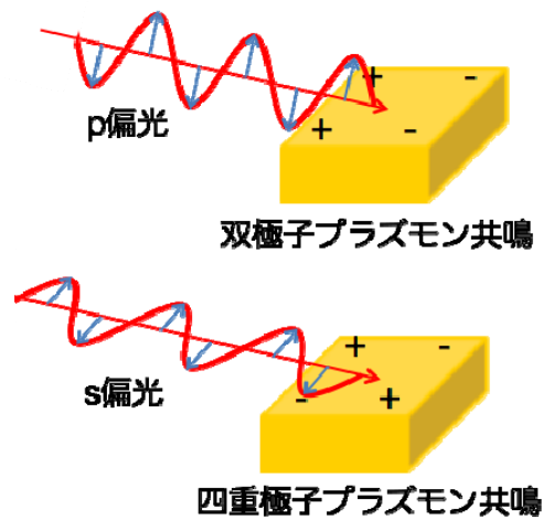
図1 入射光の波の向き（偏光）によって誘起される双極子プラズモン共鳴と四重極子プラズモン共鳴の略図。生じる+と-の位置関係により双極子と四重極子は区別される。
