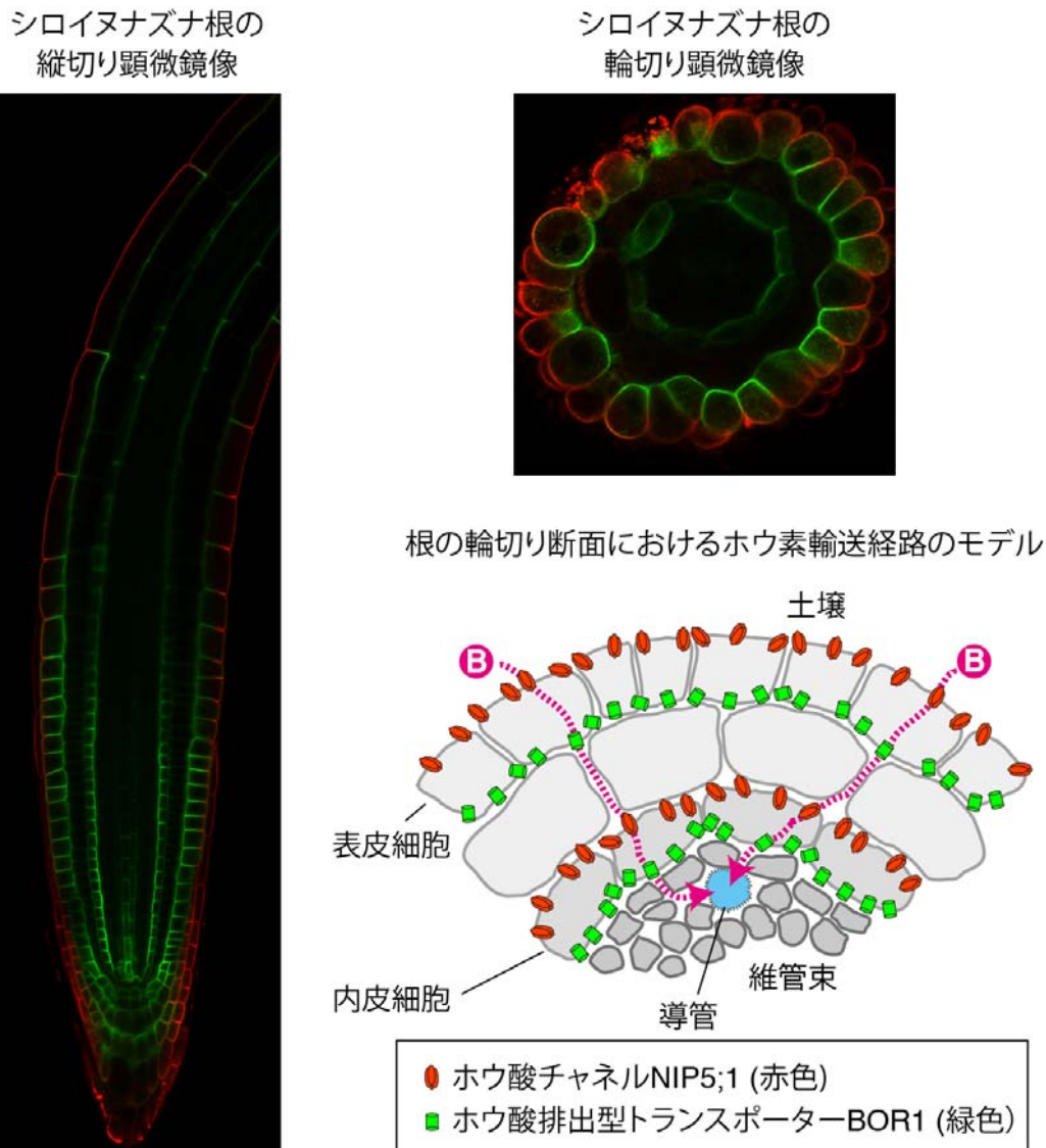
解説図 1 シロイヌナズナの根におけるホウ酸輸送経路のモデル
