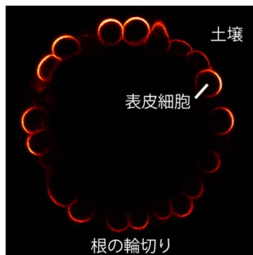
ホウ酸輸送体 NIP5;1 の局在
