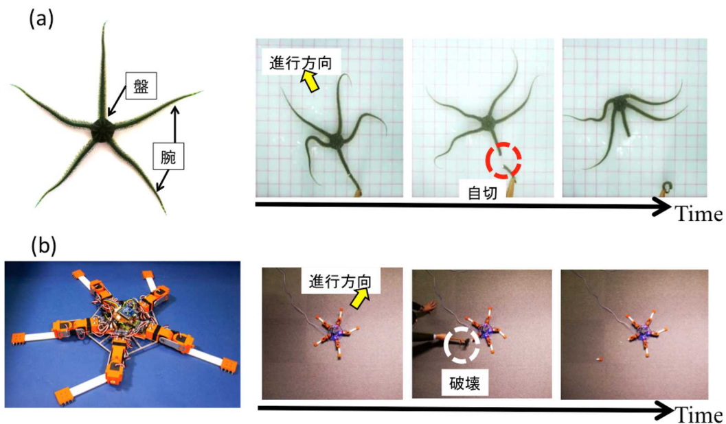
図1 (a) クモヒトデの全体像(左)と腕を自ら切断して推進する様子(右)。(b)開発したクモヒトデ型ロボット PENTABOT II(左)と、腕を破壊した時のロボットの運動の様子(右)。ロボットの腕をいかにように破壊しても即座に適応し、残った腕を協調させて推進し続けることが可能。
