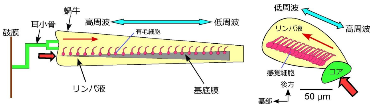
図1 ヒトの聴覚器（左。蝸牛は引き伸ばした状態）とコオロギの聴覚器（右）の原理的共通性。鼓膜の振動はヒトでは耳小骨、コオロギでは上皮コアにより液体の流れに変換される。
