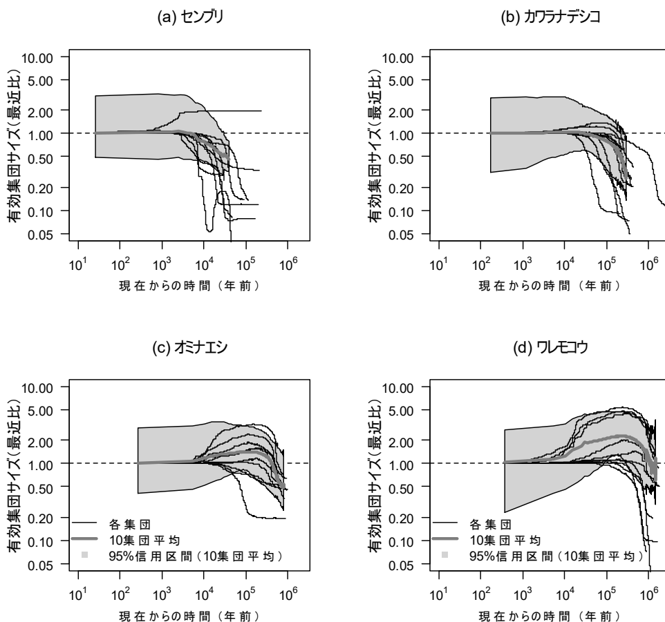
図 2. 遺伝子解析によって推測された草地性植物 4 種の集団サイズの変遷。それぞれの種について 10 カ所の草地で調査を行ない、集団サイズの変化を推測しました。横軸は現在からの時間 (右から左にかけて、過去から現在の集団サイズの変化を示します)、縦軸は数百年前の集団サイズに対する、過去の集団サイズの比率を示します。10 カ所の平均的な変遷を灰色の太線で、その 95%信用区間を灰色の区域で示しています。センブリ以外で、集団サイズは 100 万年前から 10 万年前にかけて増加し、その後カワラナ
