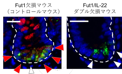
図4：IL-22はパネート細胞におけるFut2由来のフォーカスを誘導する。（緑色：パネート細胞特異的マーカーのライソザイム、赤色：フォーカス、赤矢印：Fut2 + パネート細胞、白矢印：Fut2 - パネート細胞、スケールバー：20μm）
