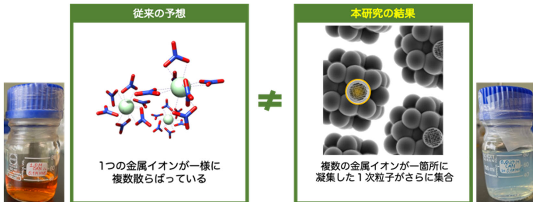
図1. セリウムの溶液モデルの比較
