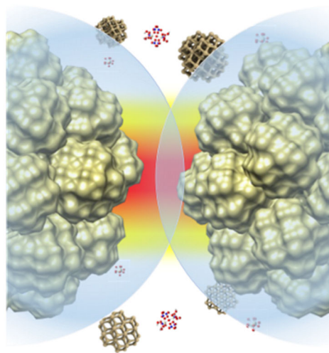
図2. 2次粒子の界面モデルとイオンの薄層
