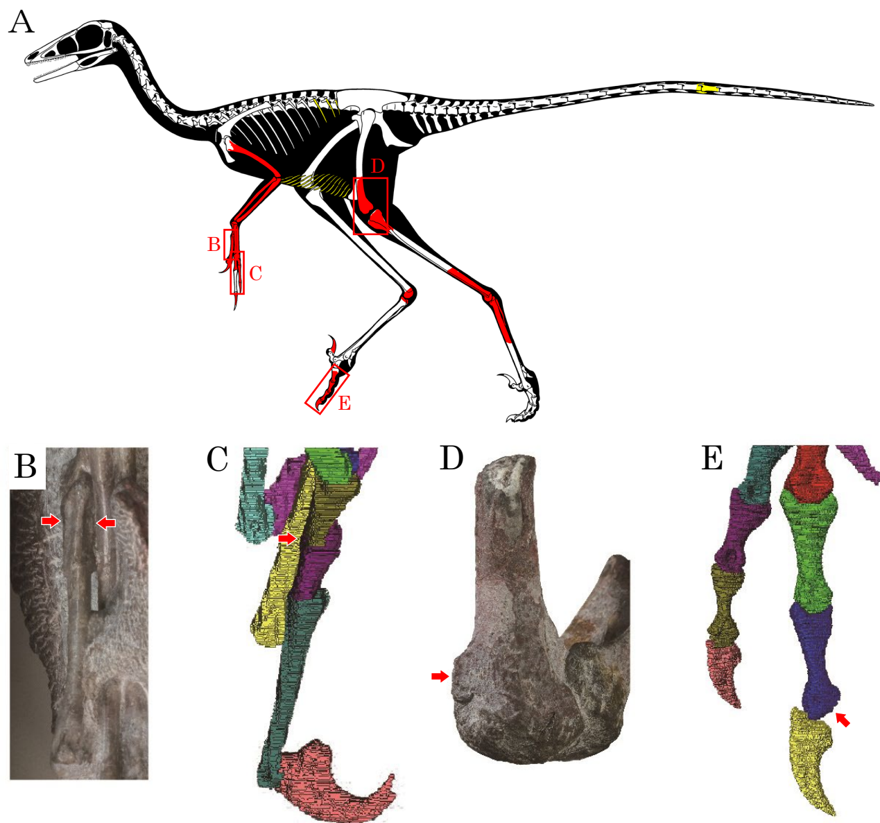
図3 ヒプノヴェナトルの全身復元骨格 ©増川玄哉（A；赤色の部分：確実な位置が分かる骨、黄色の部分：想定される骨の位置 [腹部と尾部]；スケールは1メートル）と固有の特徴（B－E）。前あしの指骨 I-1 の基部上面に1対の窪みがある（B）、前あしの指骨 III-1 と固く関節するための長い上方と下方の基部リップをもつ指骨 III-2 がある（C）、大腿骨の基部前面に遠位-近位方向に伸びる稜がある（D）、広く膨らんだ遠位腹側の縁をもつ後ろ足の指骨 III-3 の歪んだ遠位顆頭（E）
