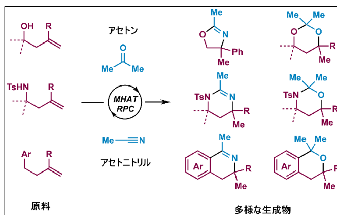
図 2. 本研究で合成した化合物群
