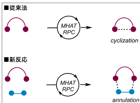
図 1. 従来法と新反応のイメージ図
