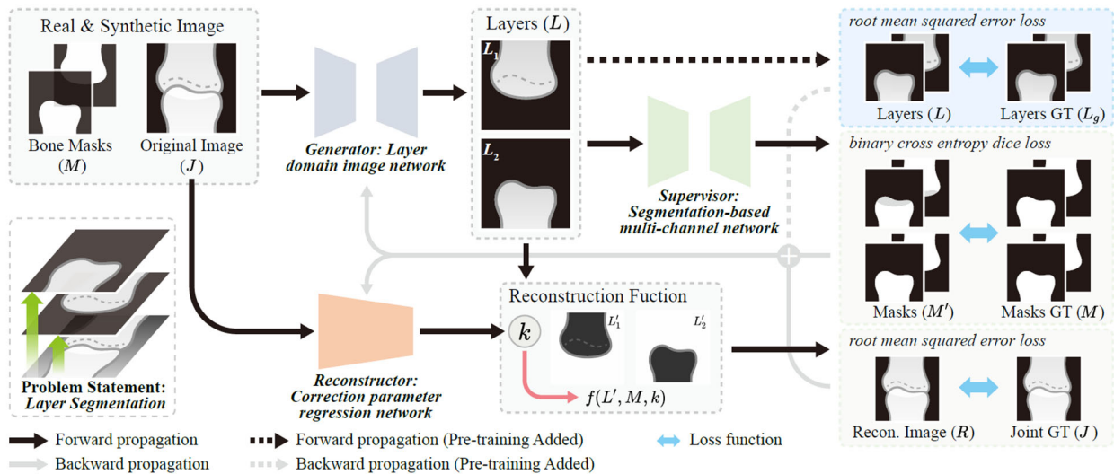
図 2. 研究開発した AI フレームワーク Bone Layer Separation GAN (BLS-GAN)
