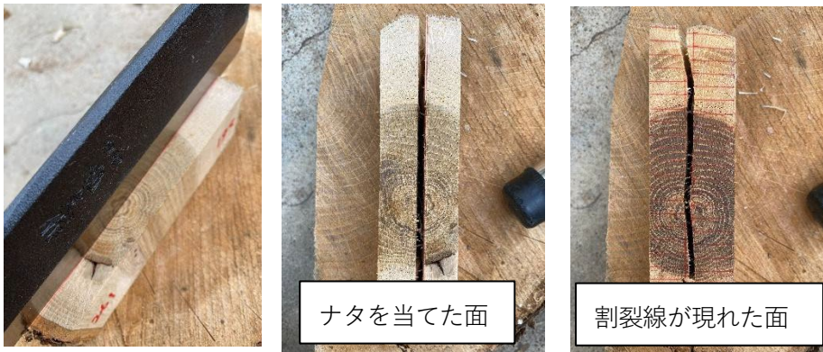
図3. 割裂法の様子。サンプルの木口面（表裏）に平行に引いた基準線にナタを当て、繊維に沿って割る。繊維が傾斜した部分の割裂線は、基準線からずれて現れる。ずれの大きさが、材のねじれの大きさを表す。
