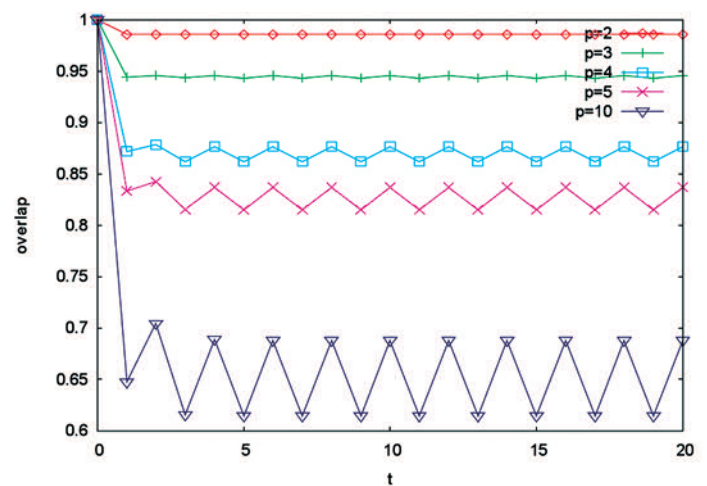
右図のような複雑ネットワーク上で定義された連想記憶における記憶パターンとニューロン状態との重なり時間の時間発展
